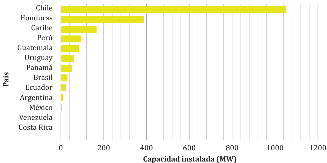
Figura 4. Capacidad instalada por país de energía solar a 2015.
