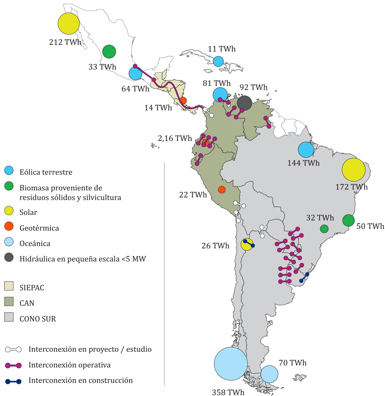
Figura 11. Mapa de ALC, indicando los tres bloques de interconexión regional (SIEPAC, CAN y Cono Sur), las interconexiones que existen en la región y ejemplos de sitios ricos en recursos de energía renovable para generación eléctrica.
