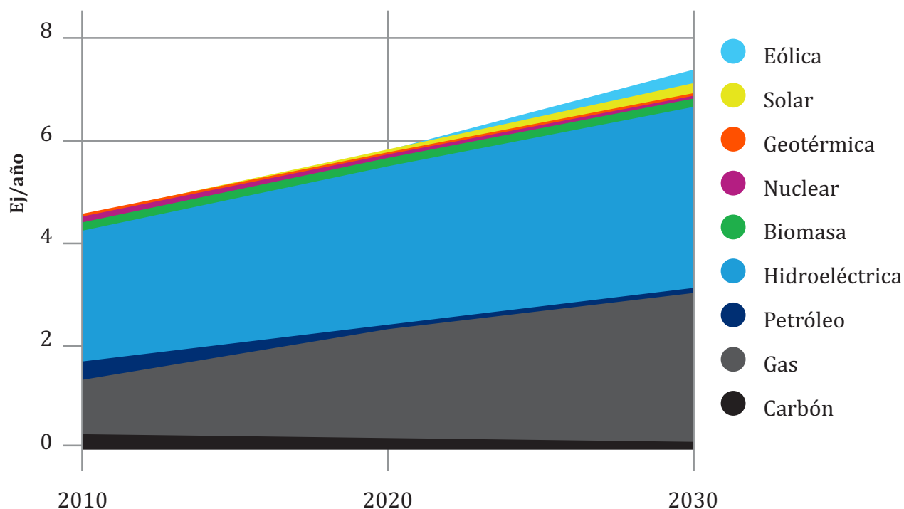
Figura 10. Evolución proyectada de la matriz eléctrica de ALC hasta 2030
