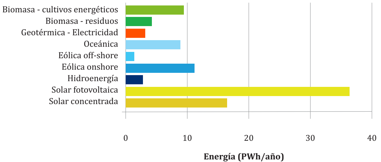
Figura 8. Potencial técnico regional total para las tecnologías renovables a largo plazo.
