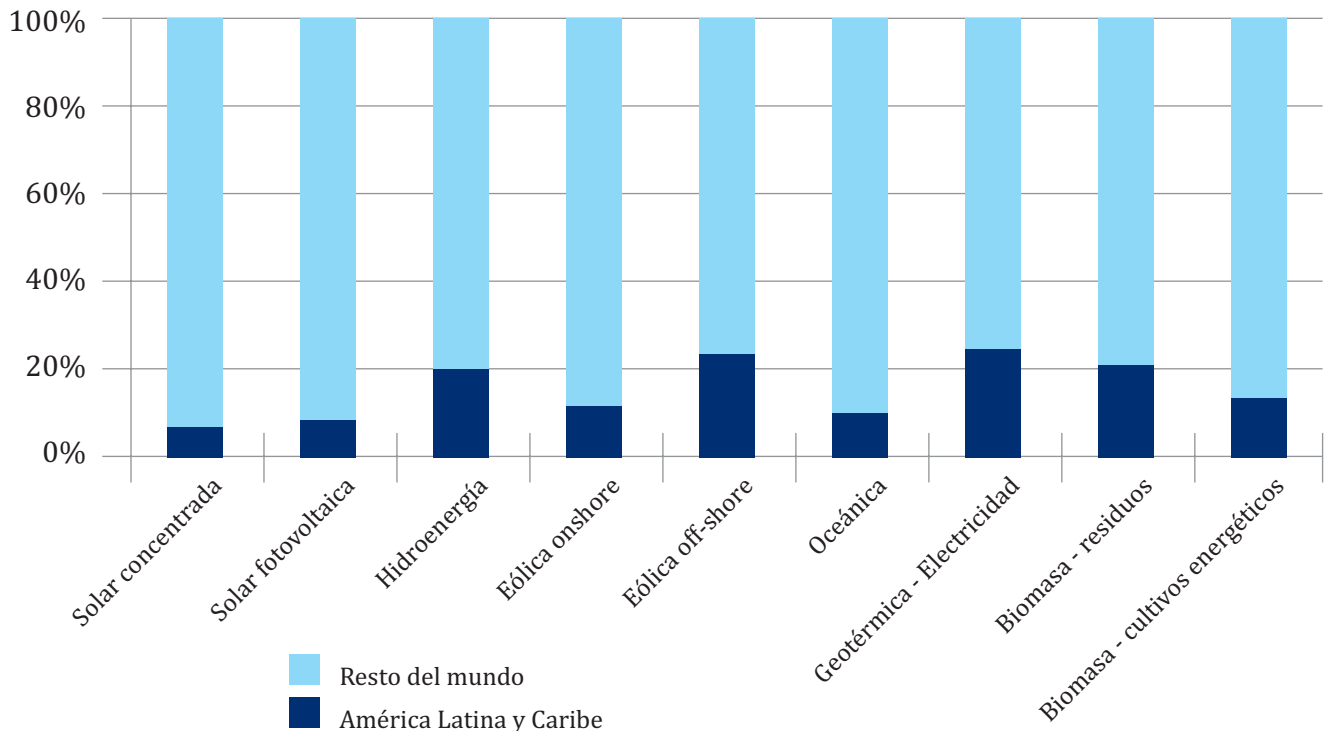
Figura 9. Porcentaje de potencial técnico de renovables en la región frente al del mundo.
